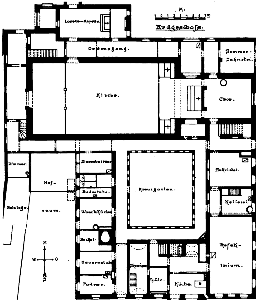
Bild 15. Grundriß des Kapuzinerklosters in Türkheim (zu S. 210).
